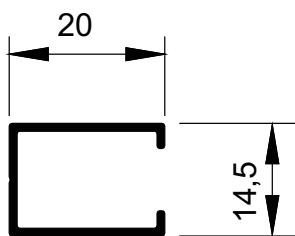
MG20-1625 0,154 kg/m
