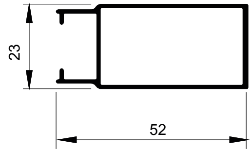
MG20-2210 0,435 kg/m
