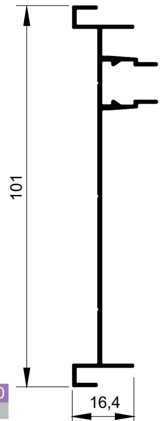
MG20-1030 0,650 kg/m
