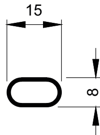
MG16-350 0,097 kg/m
