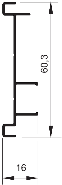
MG16-120 0,279 kg/m
