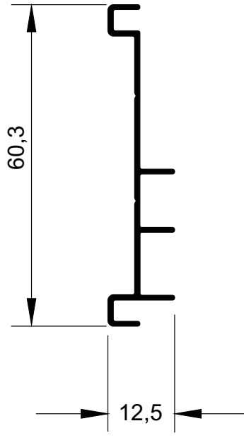
MG16-130 0,259 kg/m
