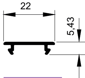
MG20-1630 0,106 kg/m
