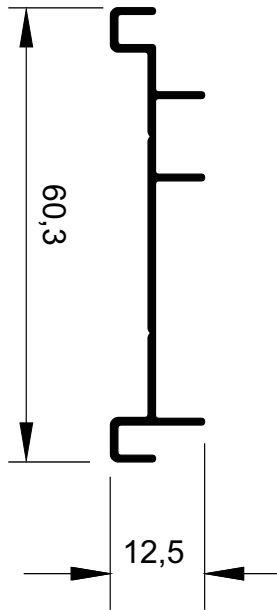
MG16-125 0,259 kg/m
