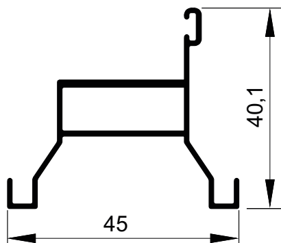
MG20-2200 0,412 kg/m
