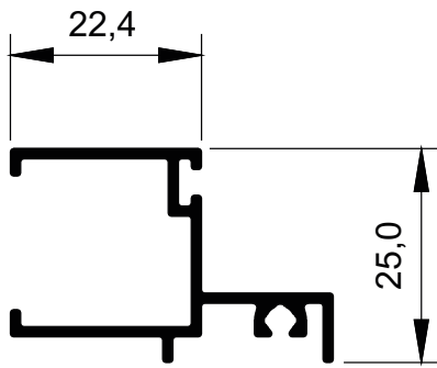
MG20-1610 0,408 kg/m
