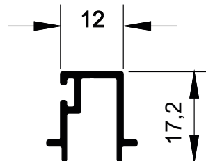
MG16-340 0,172 kg/m
