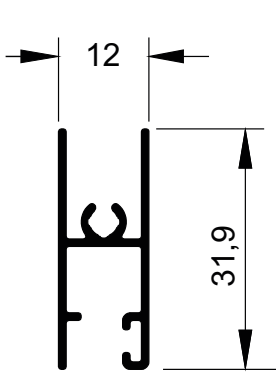
MG16-165 0,255 kg/m
