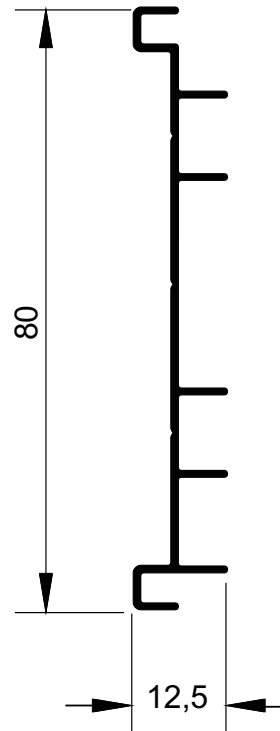
MG16-145 0,344 kg/m
