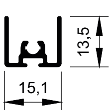
MG16-550 0,155 kg/m
