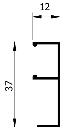
RA-347 0,197 kg/m
