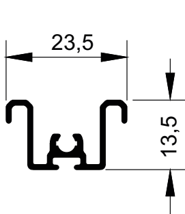
MG16-315 0,181 kg/m
