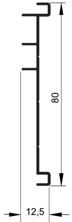
MG16-288 0,320 kg/m
