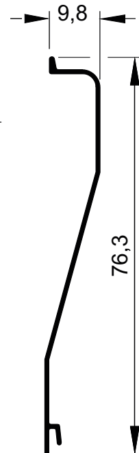
MG16-370 0,219 kg/m
