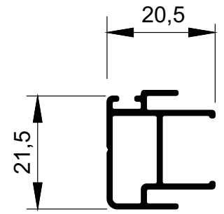
MG16-170 0,261 kg/m
