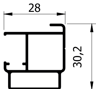
MG16-385 0,384 kg/m
