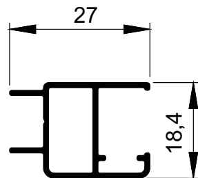
MG16-180 0,251 kg/m
