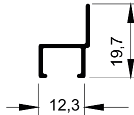
MG16-325 0,112 kg/m
