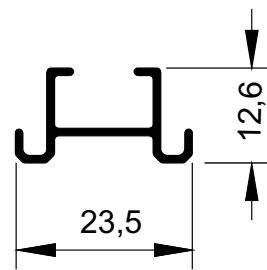
MG16-305 0,154 kg/m
