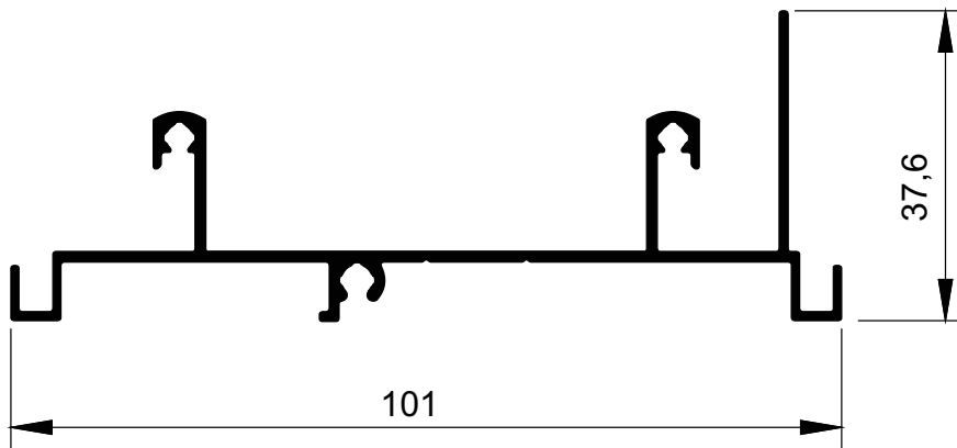
MG20-1015 0,765 kg/m
