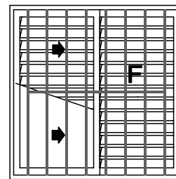
JANELA DE CORRER 3 FOLHAS 1FX 2M CG VENEZIANA
