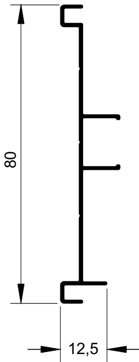
MG16-135 0,332 kg/m
