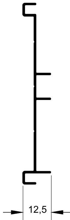
MG16-140 0,312 kg/m
