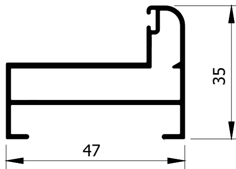
MG20-2230 0,574 kg/m
