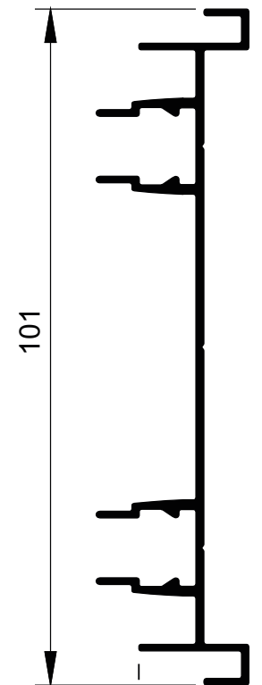
MG20-1035 0,659 kg/m
