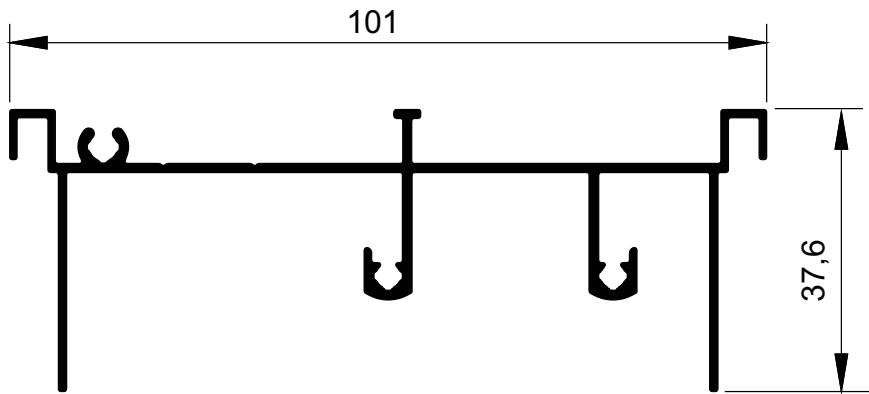
MG20-1110 0,849 kg/m
