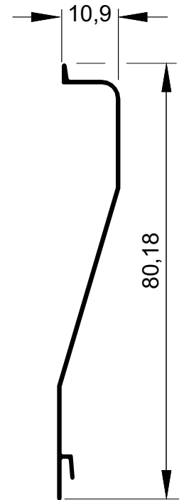
MG16-371 0,221 kg/m
