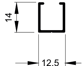
MG16-355 0,112 kg/m
