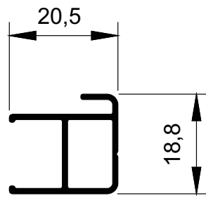
MG16-155 0,207 kg/m
