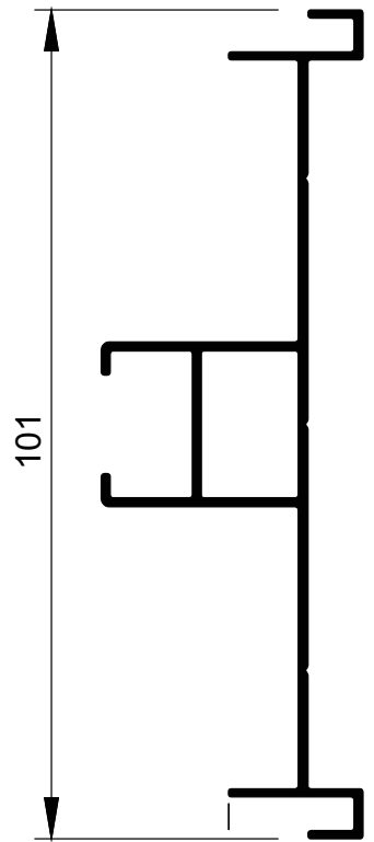
MG20-1030 0,650 kg/m
