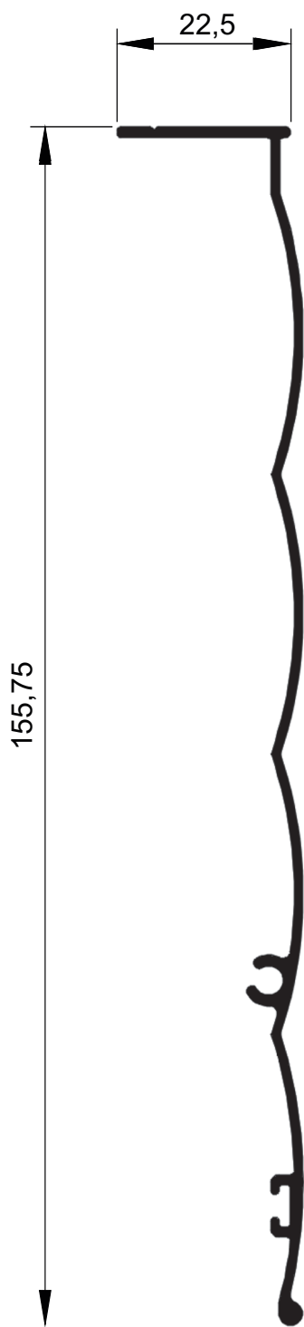
MG16-225 0,636 kg/m
