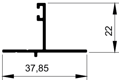
MG20-1615 0,222 kg/m
