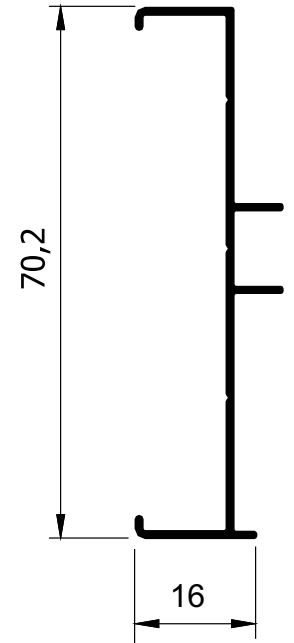
MG16-390 0,301 kg/m
