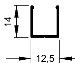
MG16-365 0,107 kg/m
