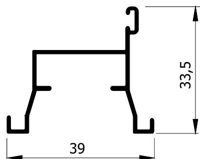
MG20-2240 0,300 kg/m
