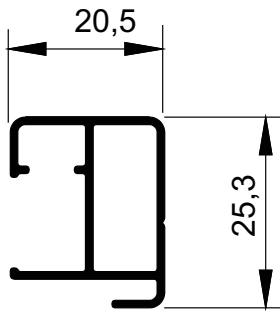
MG16-150 0,266 kg/m
