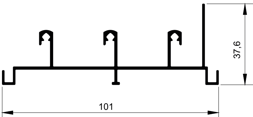
MG20-1145 0,841 kg/m
