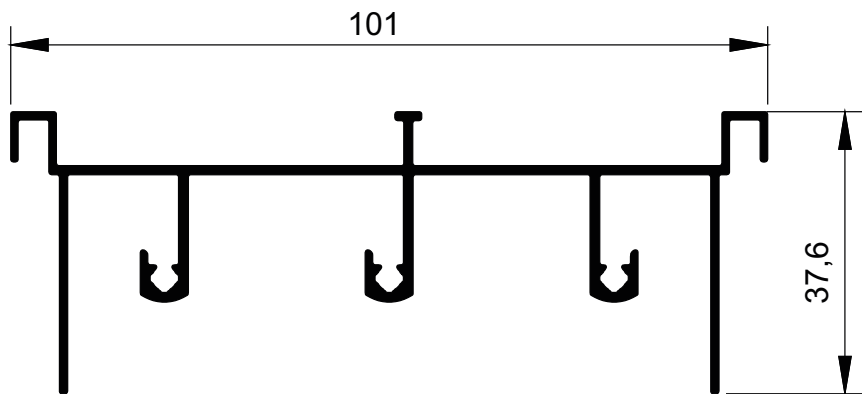
MG20-1140 0,904 kg/m
