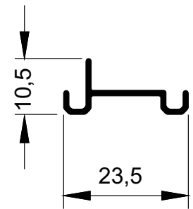
MG16-310 0,112 kg/m
