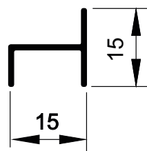
MG16-555 0,097 kg/m
