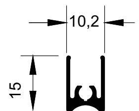
MG16-330 0,176 kg/m
