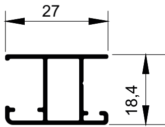
MG16-175 0,265 kg/m
