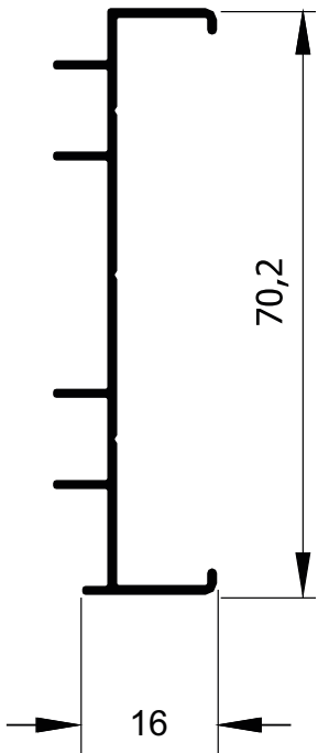
MG16-395 0,333 kg/m
