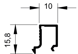
BG-035 0,119 kg/m
