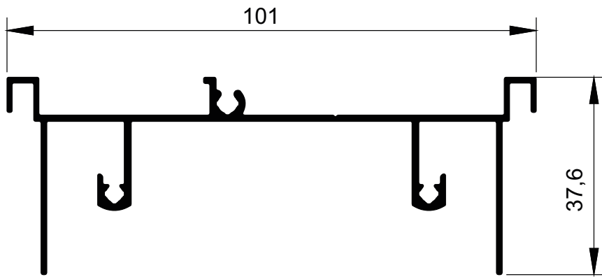
MG20-1010 0,828 kg/m
