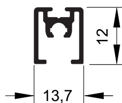
MG16-345 0,167 kg/m
