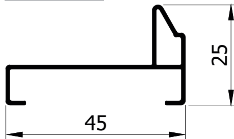
MG20-2230 0,574 kg/m
