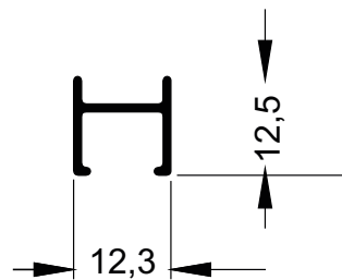
MG16-185 0,285 kg/m
