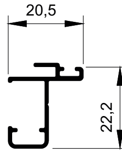
MG16-160 0,194 kg/m
