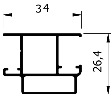
MG16-380 0,407kg/m
