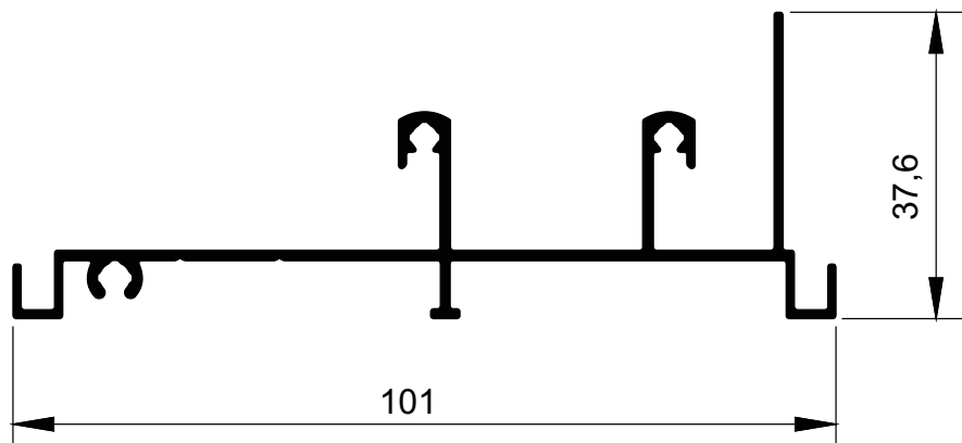
MG20-1105 0,779 kg/m
