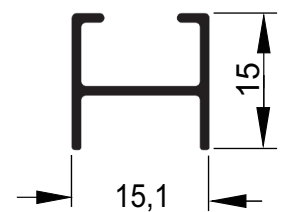
MG16-545 0,130 kg/m
