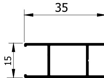
MG16-375 0,262 kg/m
