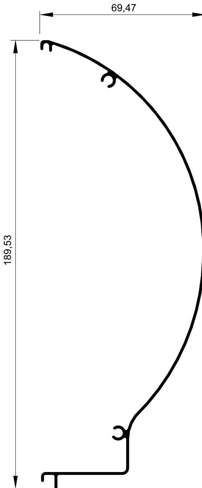
MG16-231 0,904 kg/m
