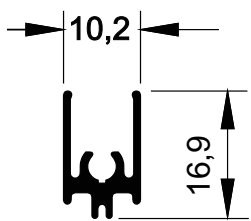
MG16-335 0,171 kg/m
